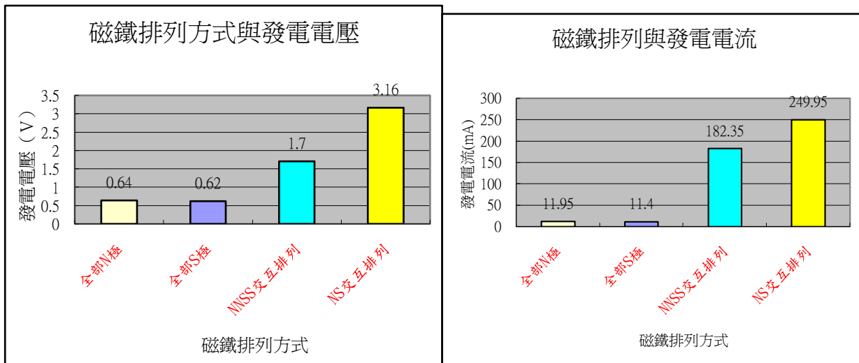
統計表一：磁鐵排列與發電電壓、電流統計表
